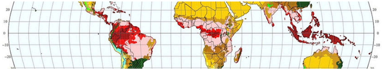
Koppen Geiger Map 1901-1925
